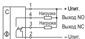
Схема подключения
