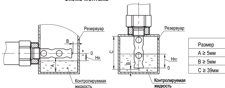
Схема монтажа
