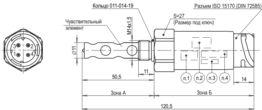
Габаритный чертеж
